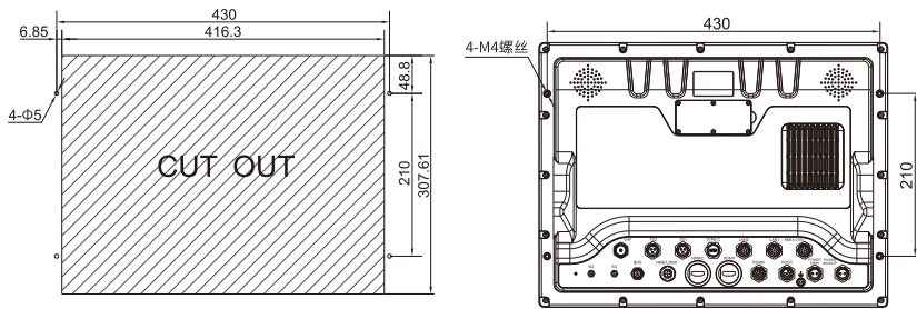
开孔尺寸图
