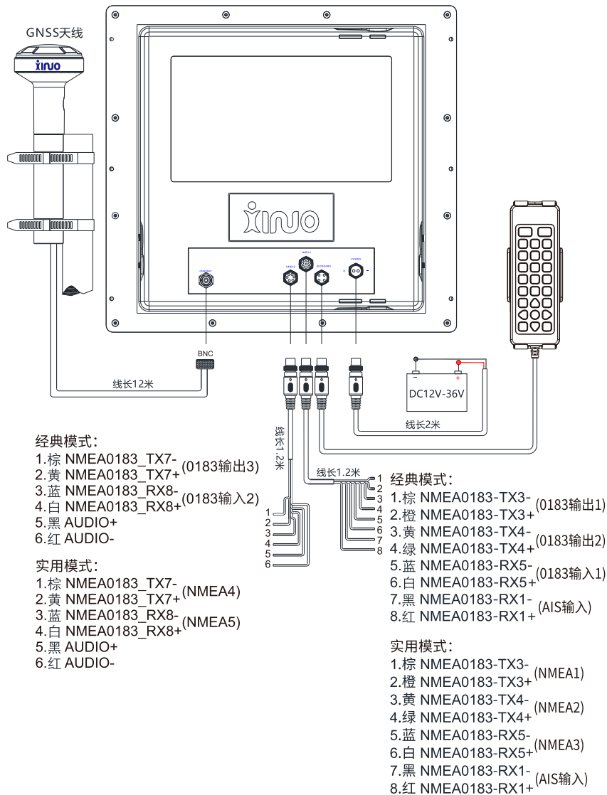
图1. HM-1817
