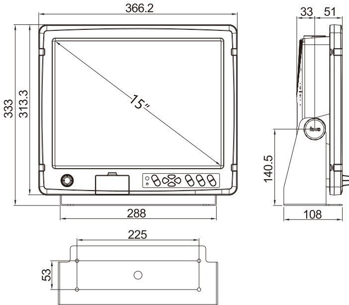
HM-1815&HM-5900(15")台面安装图 [单位:mm]
