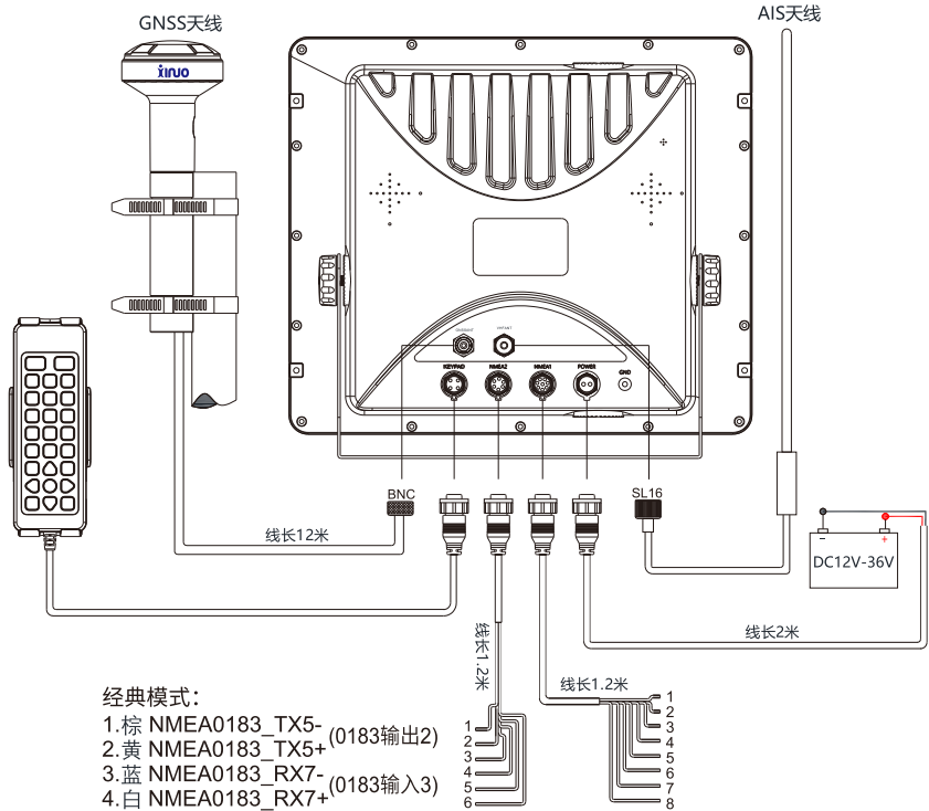
图4. HM-5900(15")
