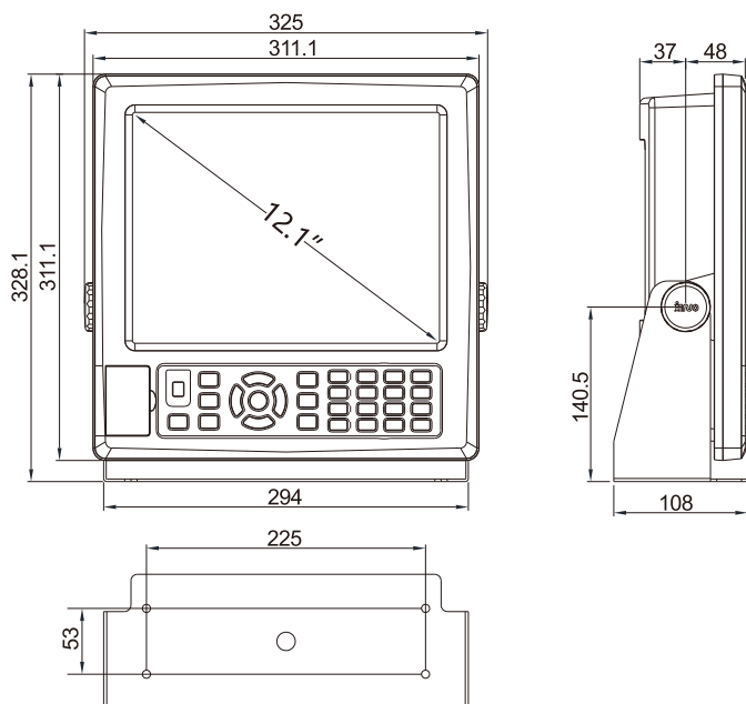
HM-1512N&HM-5912台面安装图 [单位:mm]
