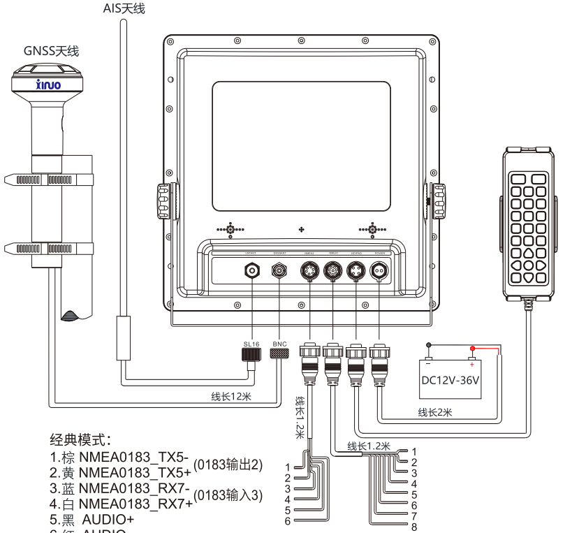
图6. HM-5912
