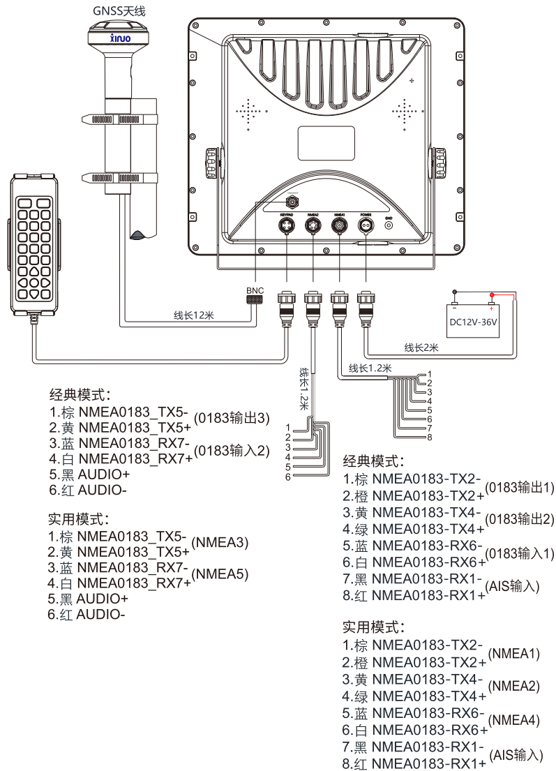
图3. HM-1815
