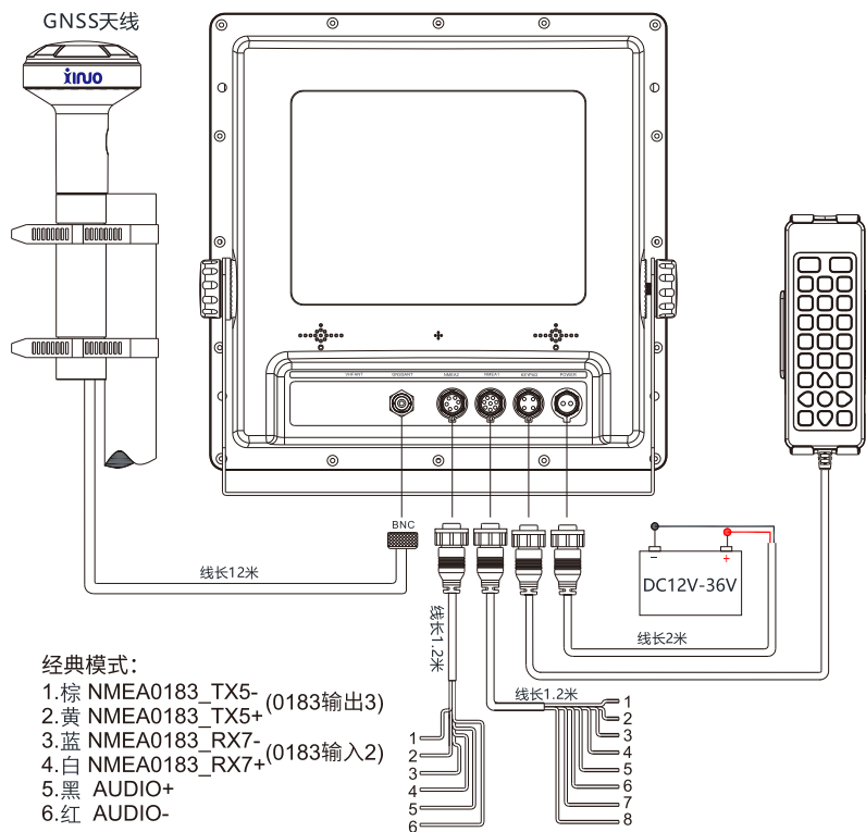
图5. HM-1512N
